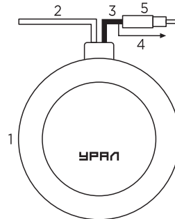
Рис. 2 Элементы антенны
