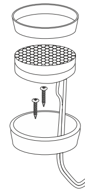
Наружная установка
