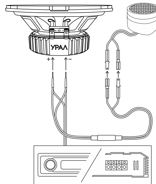
Наружная установка
