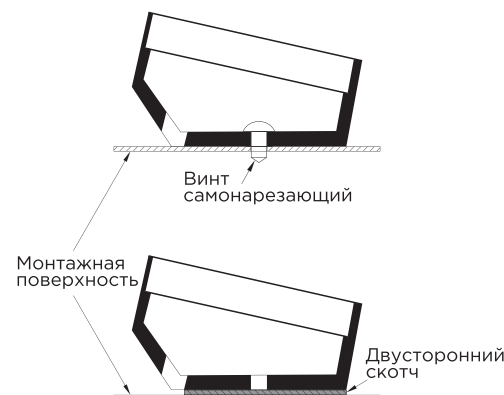
Наружный монтаж
